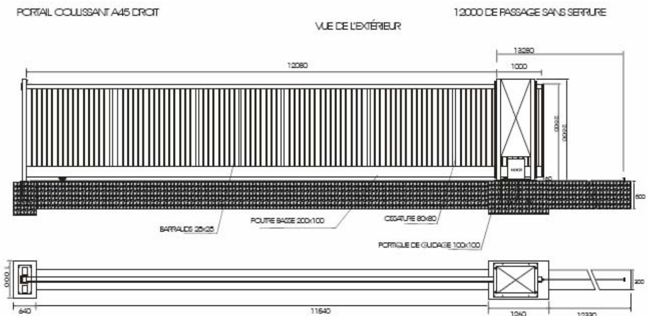
SCHEMA D'IMPLANTATION
